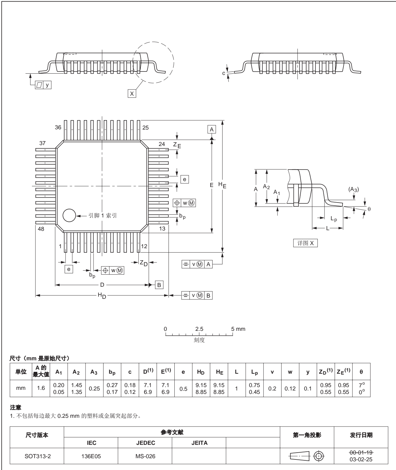
图 34. 封装尺寸 LQFP48 (SOT313-2)
