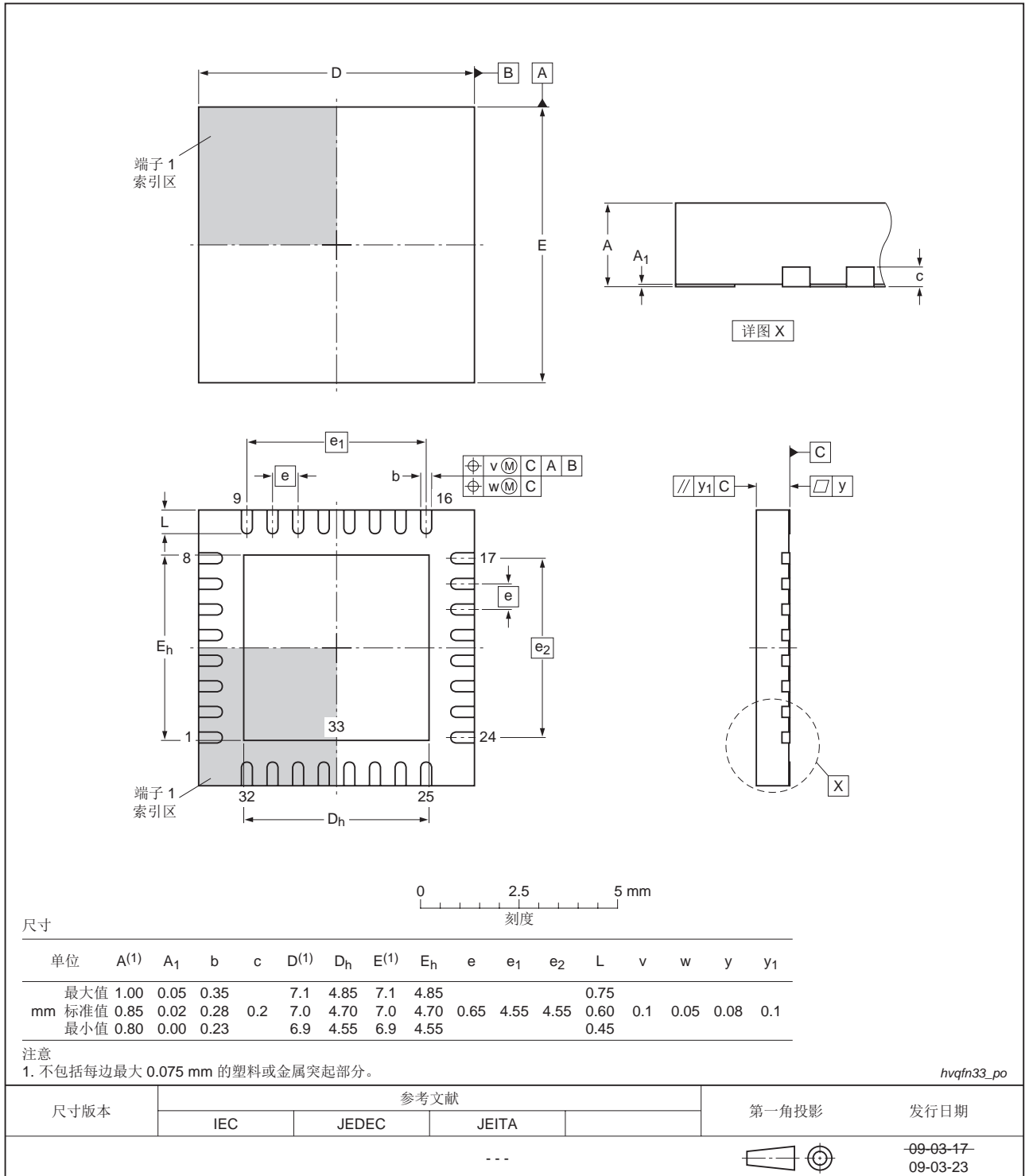
图 32. 封装尺寸 HVQFN33 (7 x 7 x 0.85 mm)
