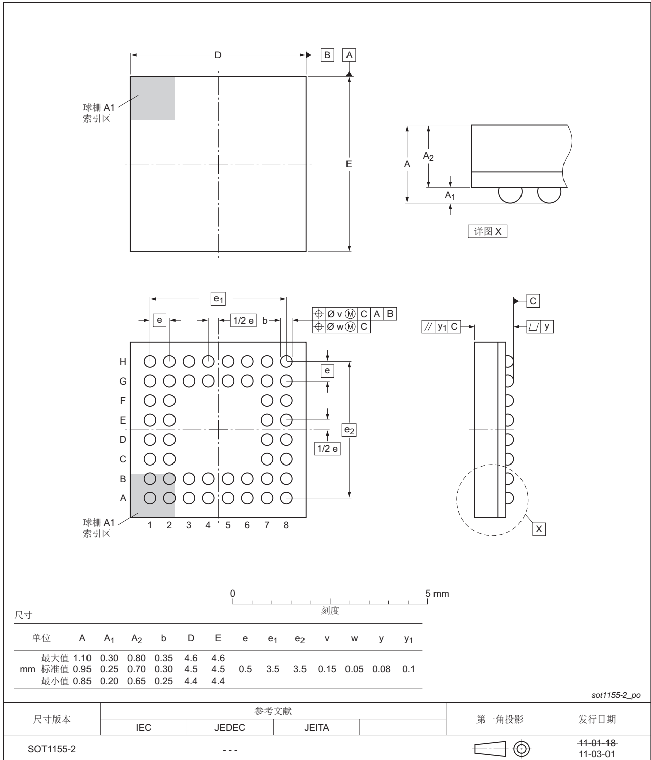
图 36. 封装尺寸 TFBGA48 (SOT1155-2)
