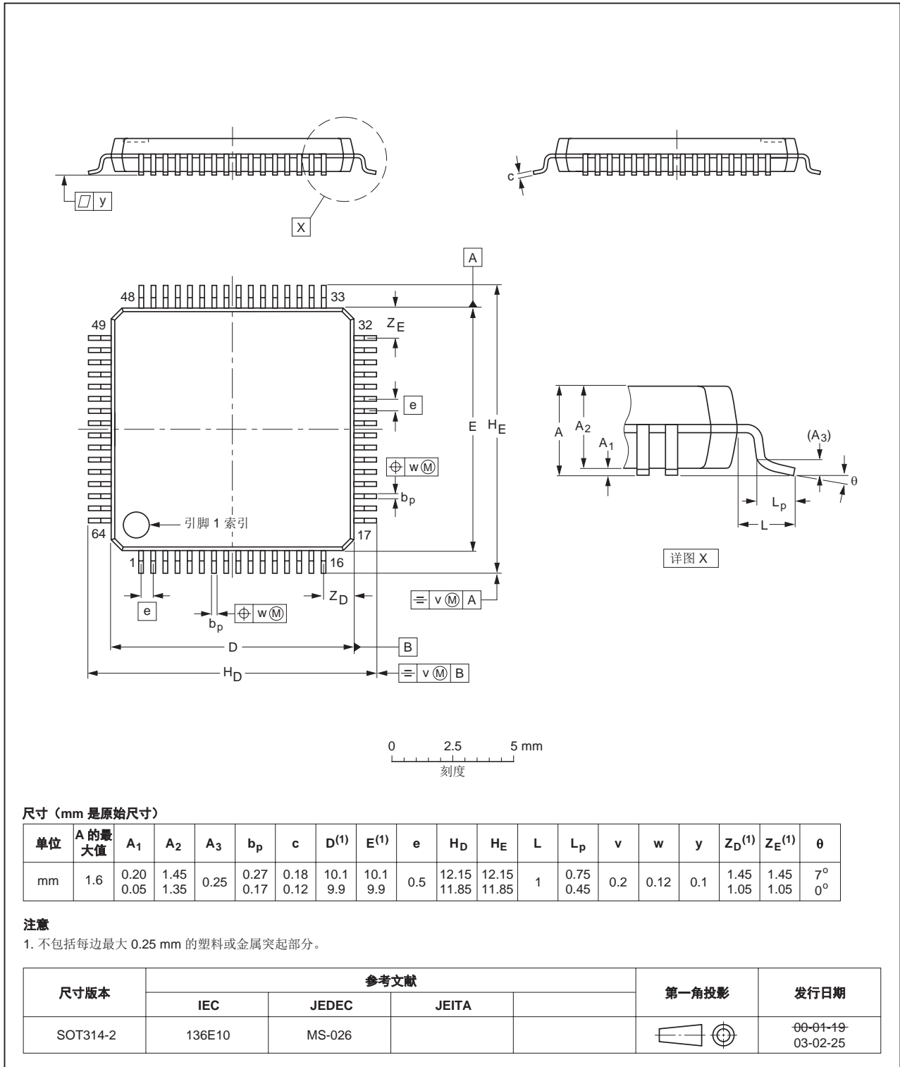
图 35. 封装尺寸 LQFP64 (SOT314-2)
