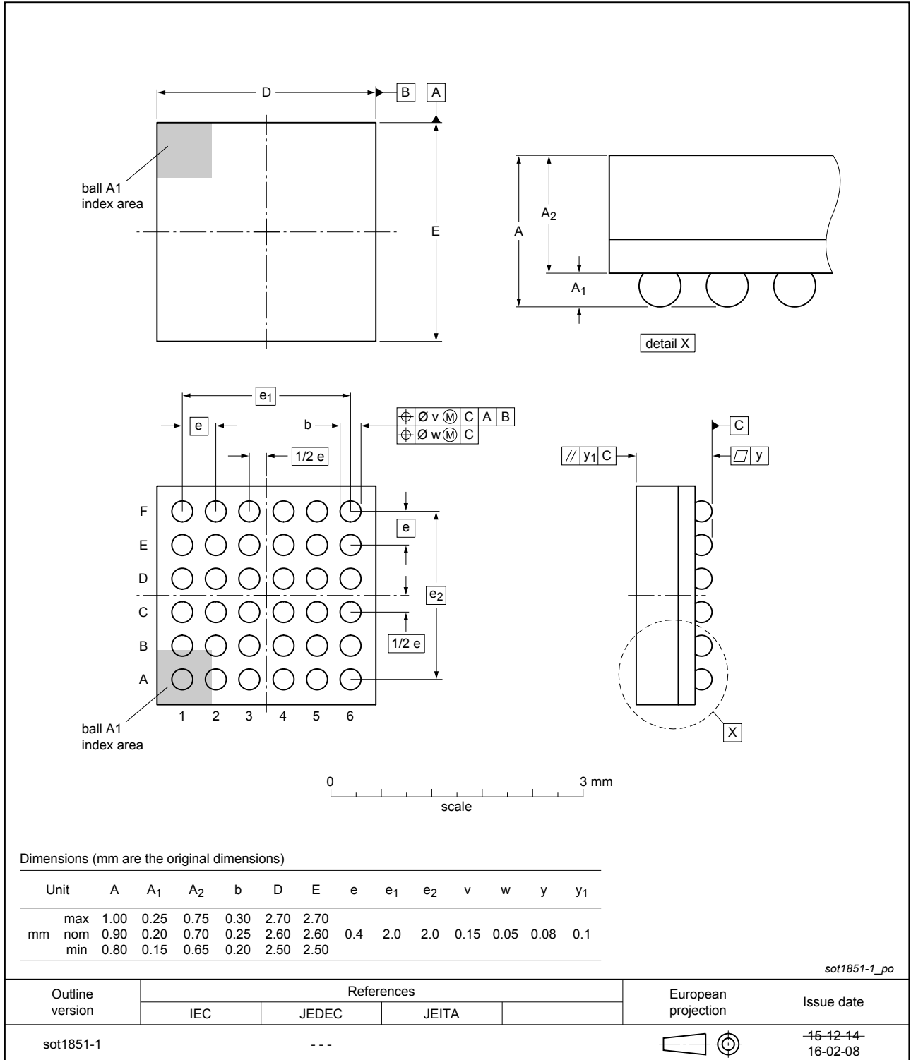
Fig. 1. Package outline VFBGA36 (SOT1851-1)
