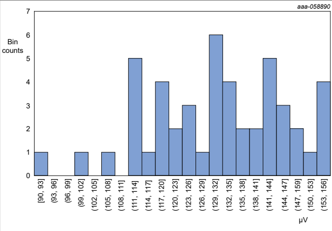
Figure 81. Vsense INL
