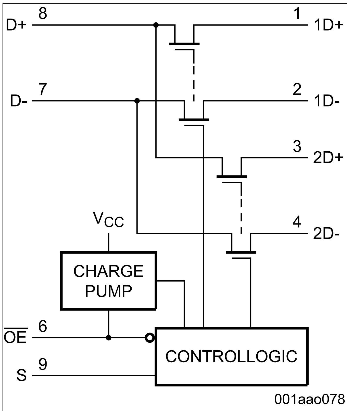
NX3DV221ブロック図 Block Diagram
